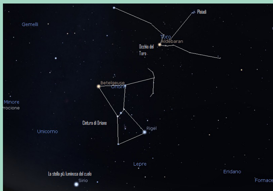
Immagine 2: Orione, il Toro, Aldebaran, la cintura di Orione, Marte, Sirio e le Pleiadi. (Stellarium)
