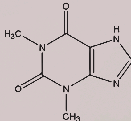
TEOFILLINA
