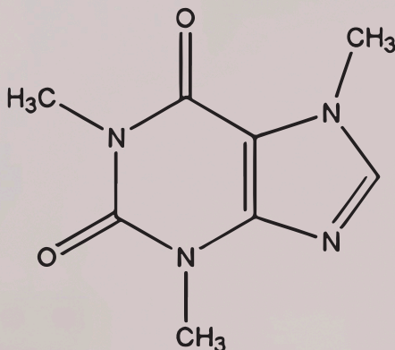
CAFFEINA
