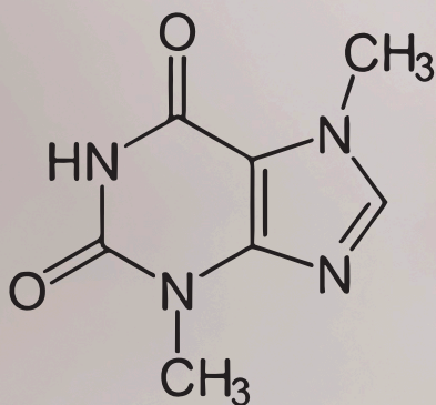
TEOBROMINA
